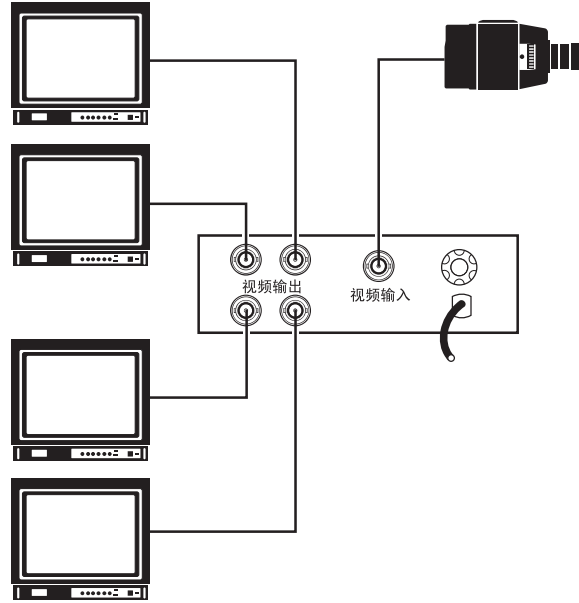
典型配置图
