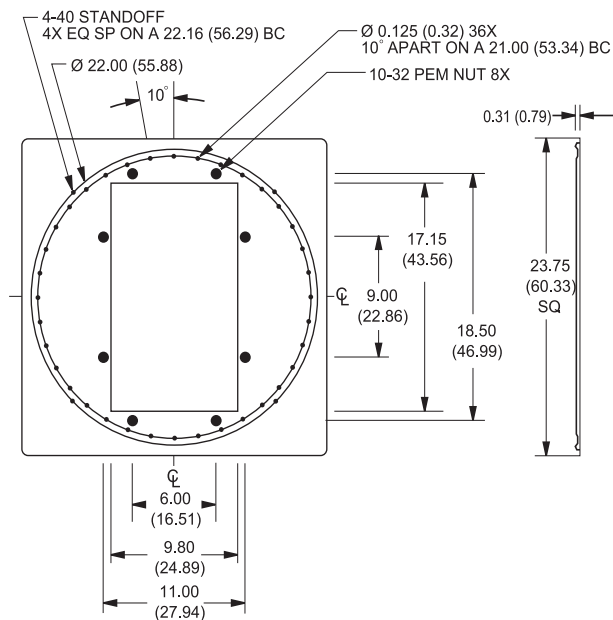
E1003 尺寸图
